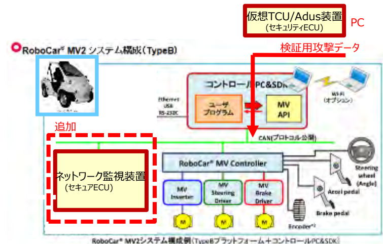
車内LANに対する評価環境 (CAN bus)
