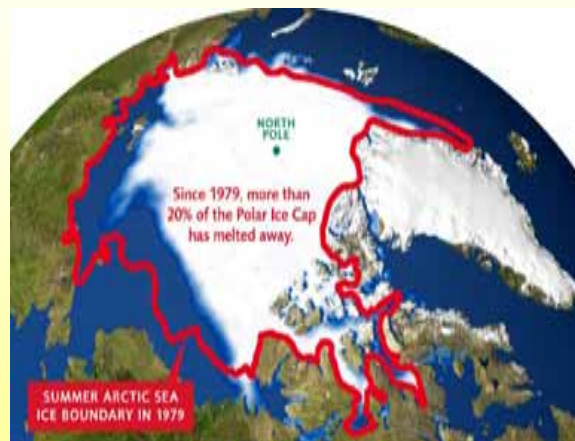
温暖化の進行による北極海の海氷の融解
