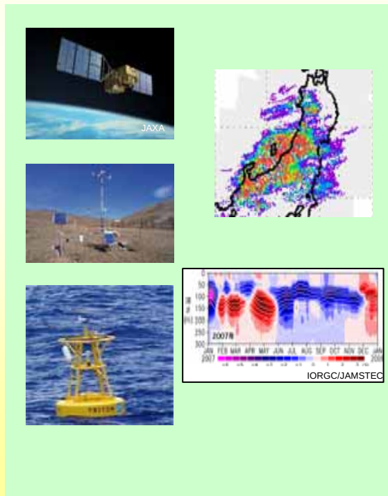
衛星、陸域、海洋からの観測
