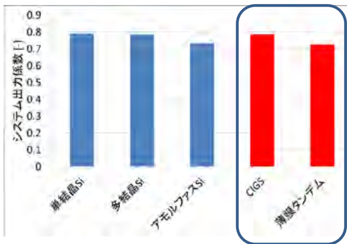
図1 太陽電池種別の発電性能比較
