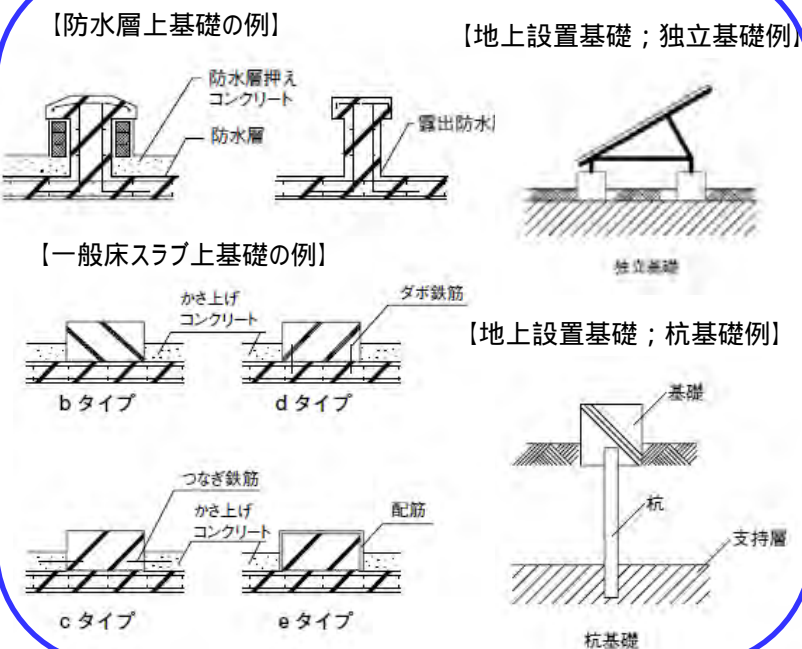
図2 基礎の分類例
