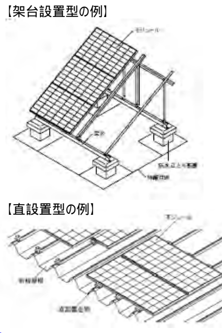
図3 架台の分類例
