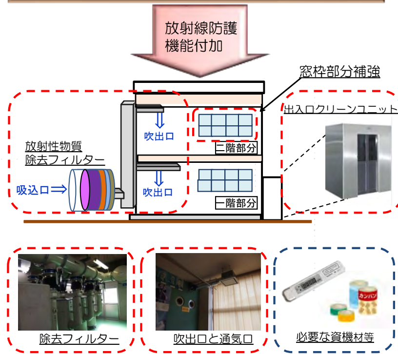
放射線防護対策のイメージ図
