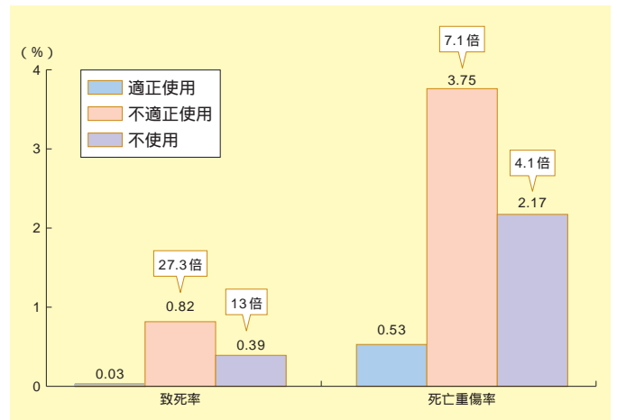
チャイルドシート使用有無別致死率及び死亡重傷率（平成21年）
