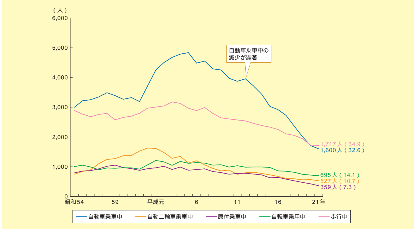
状態別交通事故死者数の推移
