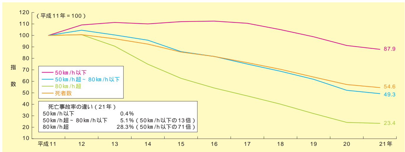
危険認知速度別交通事故件数(一般道路)及び死者数の推移
