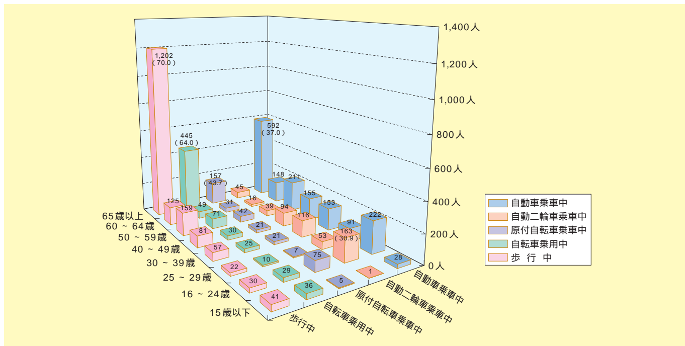
平成21年中の状態別・年齢層別交通事故死者数
