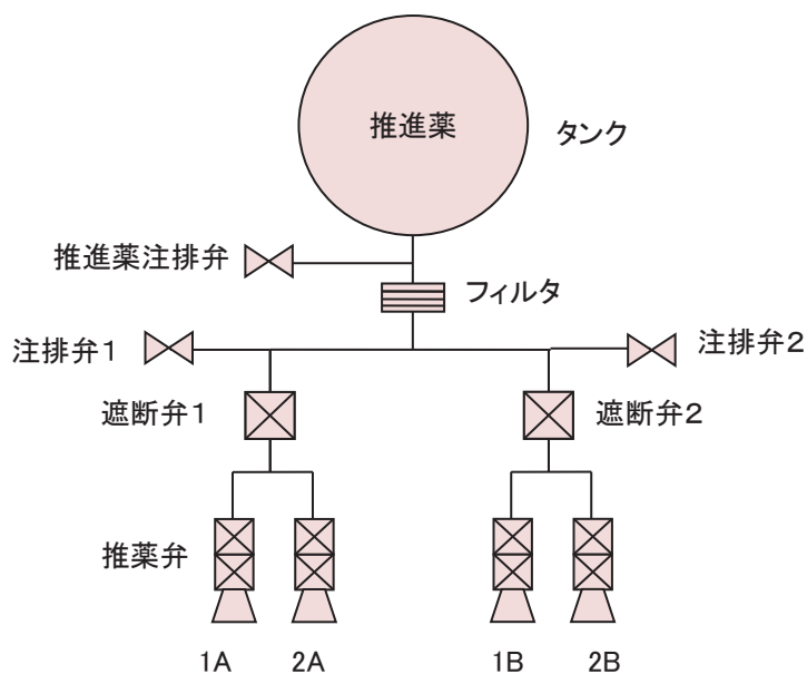
図 3.1-1 推進系構成図
