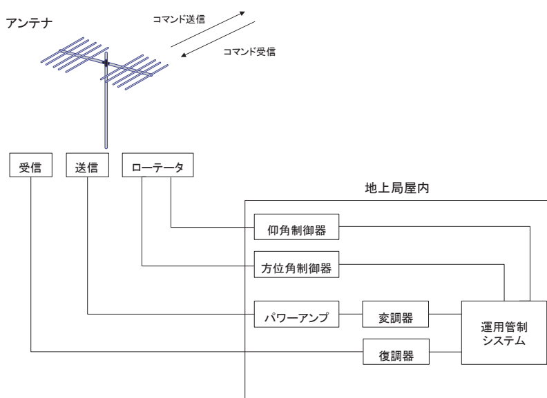
図 2-1 地上局××× 構成図
