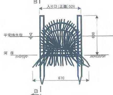
正面図
