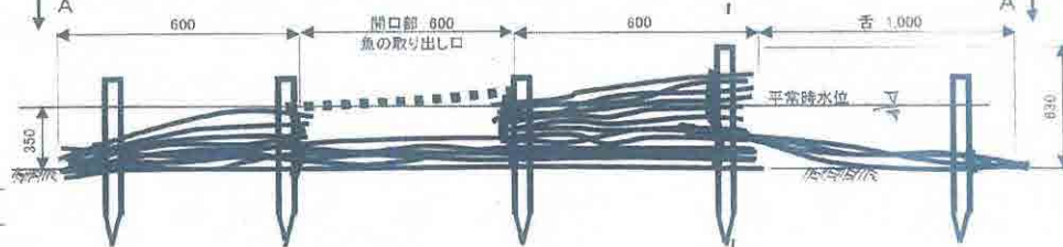
正面図
