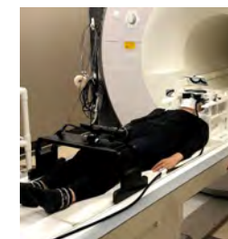
広視野fMRI用視線計測システム試作機
