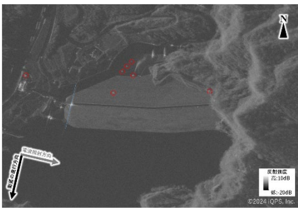
図-1 小型衛星の堤体観測結果 （強度画像 QPS-SAR Spotlightモード）
