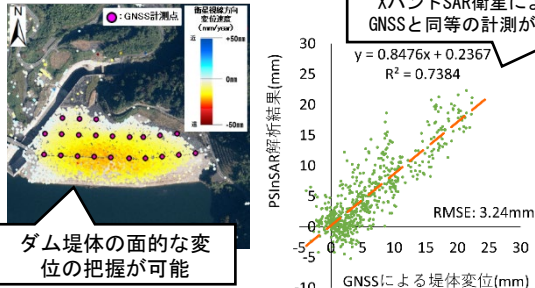
図-3 ダム堤体変位実測データとの比較
