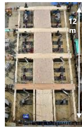
設計ガイドライン案作成のための実験（林野庁事業）
