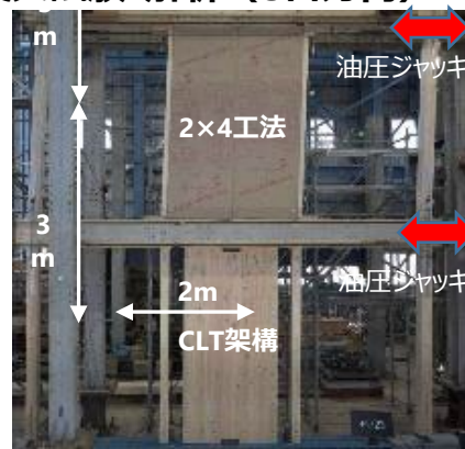
CLT+2×4工法架構の実大実験
