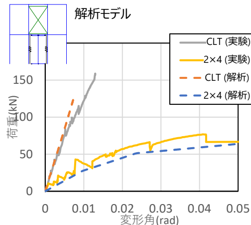
実験結果のシミュレーション
