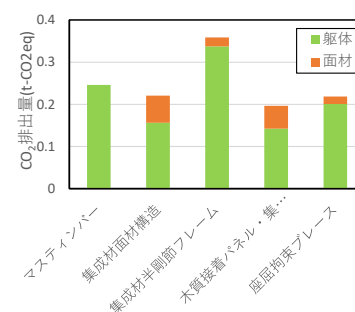
床面積当たりのCO 2 貯蔵量
