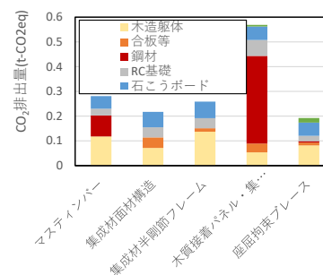
床面積当たりのCO 2 排出量
