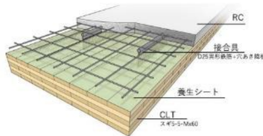
CLT合成床構造の構成
