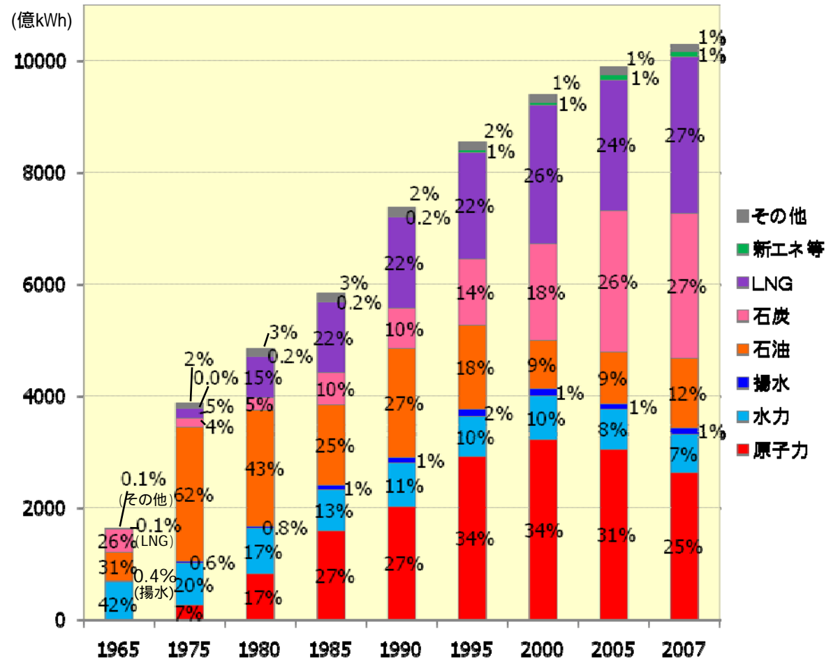
発電電力量の推移 (一般電気事業用)
