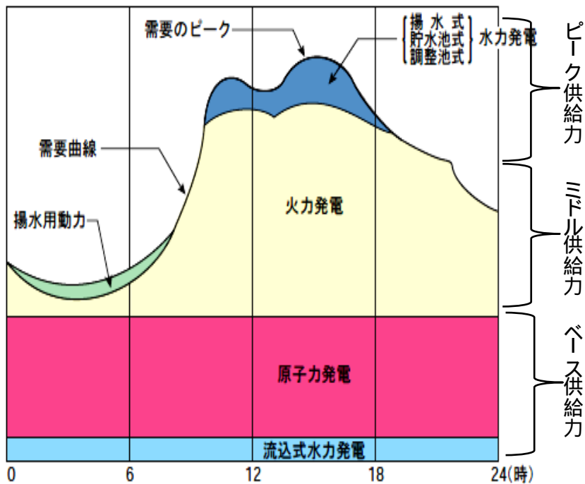
1日の電力需要と供給構成
