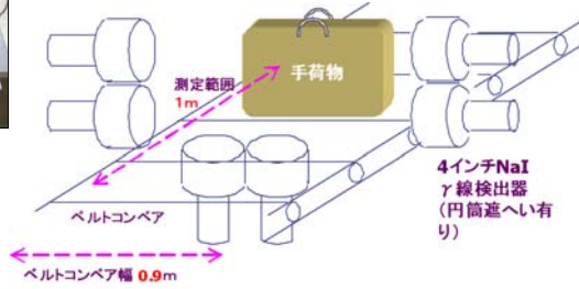
図 8 コバルト 60 等放射性物質の検出実験及びシミュレーション体系
