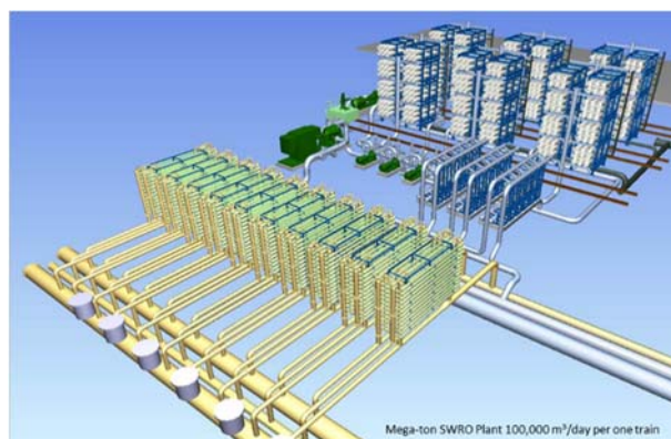
図 2. メガトンプラント（1系列）のイメージ図
