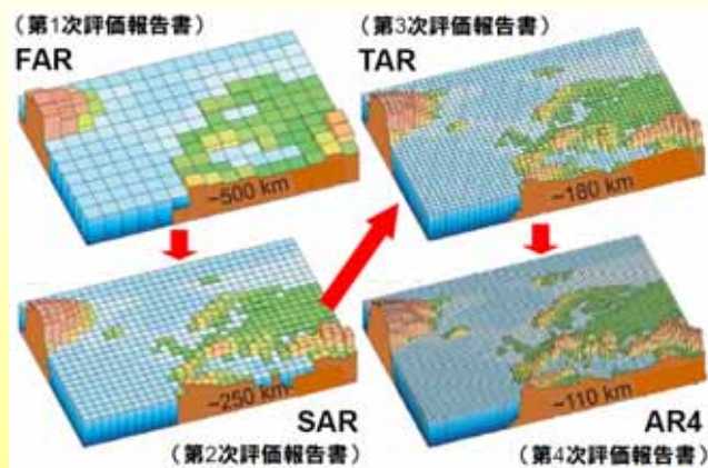
IPCC報告書が用いた気候モデルの解像度 ~ FAR, SAR, TAR, AR4 ~
