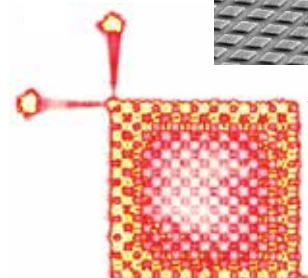
トポロジカルなフォトリック結晶 21
