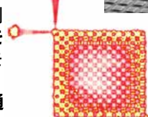
トポロジカルなフォトニック結晶 7
