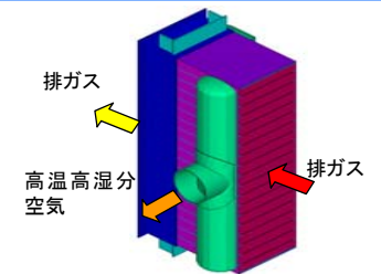
再生熱交換器ブロック概略図
