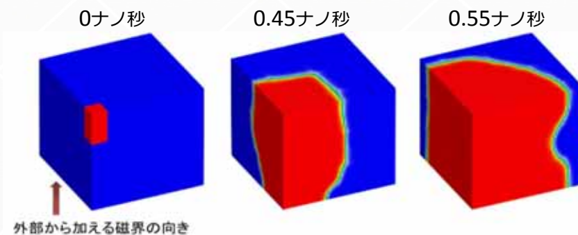
図：多結晶モデルの磁化反転シミュレーション
