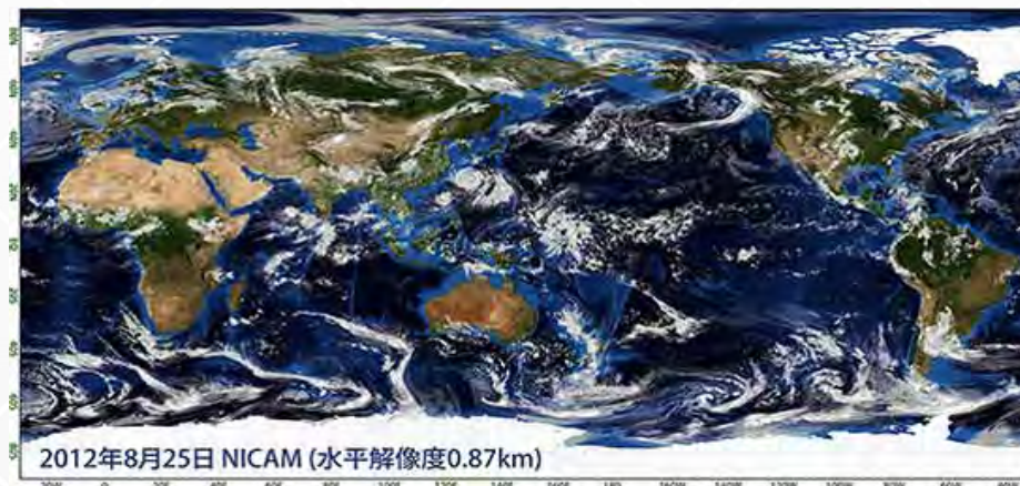
図：2012年8月25日12時(世界標準時)の全球の雲分布
