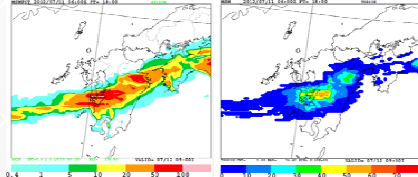
(図3)アンサンブル予報による最大降水量の分布図
