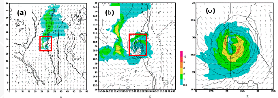
図2. (a)(b)「京」を用いて再現したあるメンバーの高度20mの雨水量(g/kg)と水平風分布、(c)風速(m/s)。数値モデルの水平解像度は50m。 (b),(c)それぞれ(a)と(b)の赤枠内の拡大図。
