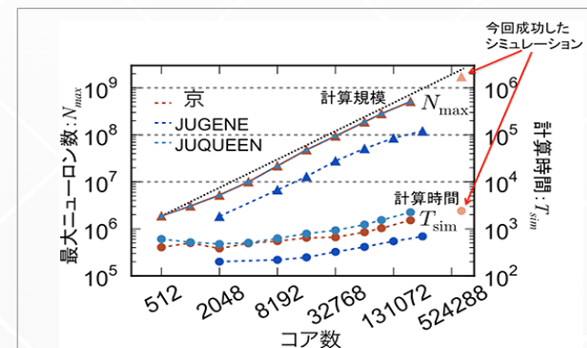
図: JUQUEEN によるNESTと「京」によるNESTのシミュレーション結果の比較
