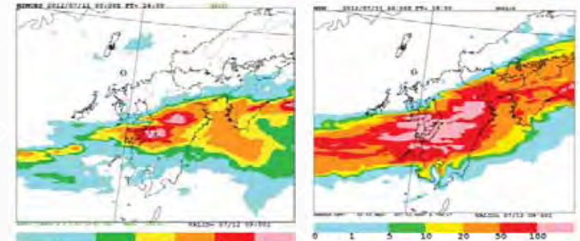
(図2)前日15時を初期値とするスーパーコンピュータ京による予測
