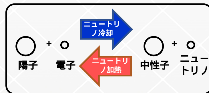
ニュートリノができる反応と 無くなる反応
