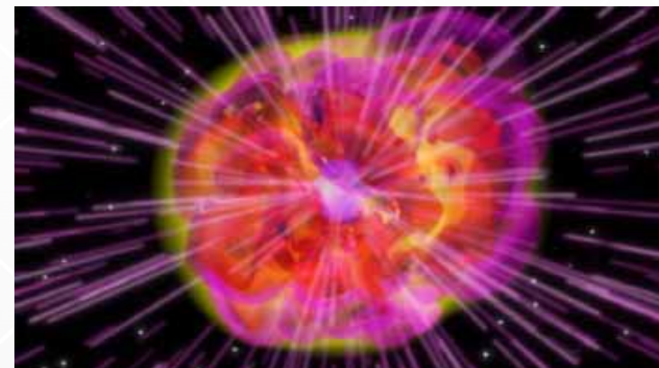
超新星爆発のイメージ図 (国立天文台プレスリリースより)
