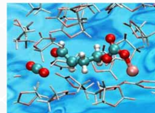
図：EC溶媒中の重合反応の最終生成物 ⇒添加剤導入時のSEI形成の素材となる
