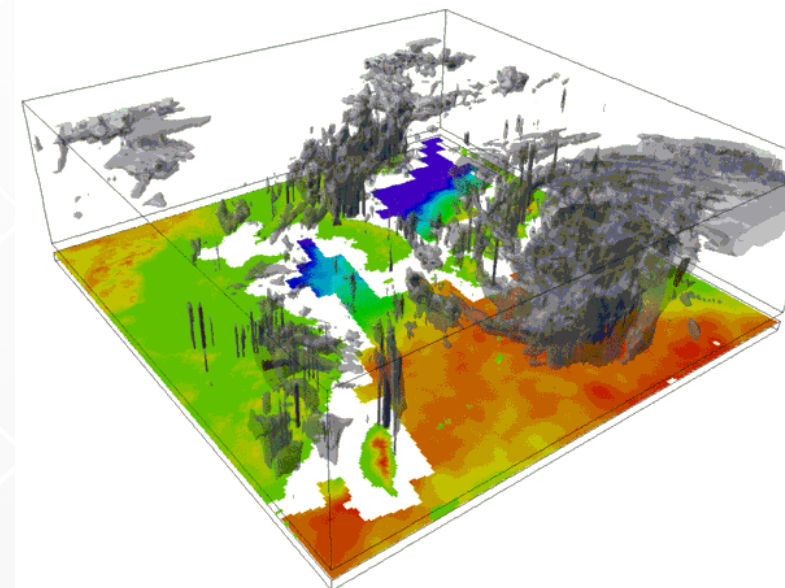
2012年台風第15号の通過に伴う海面水温の低下 (JAMSTECプレスリリースより) 計算の初期時刻は2012年8月25日21時(日本時間)
