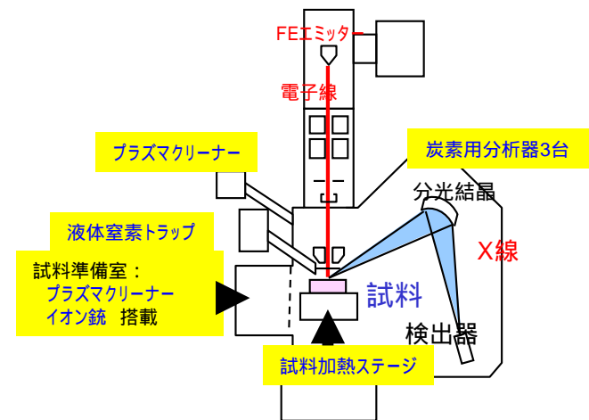
完成したC量評価装置
