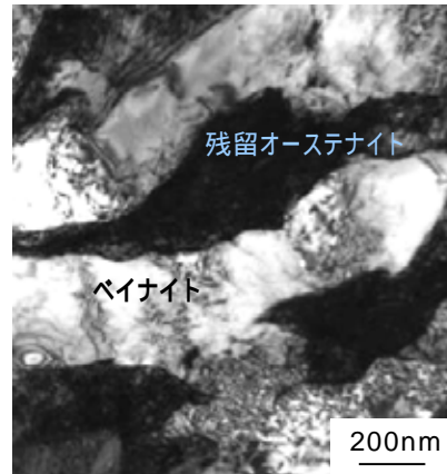
達成した高強度鋼伸び鋼板の組織
