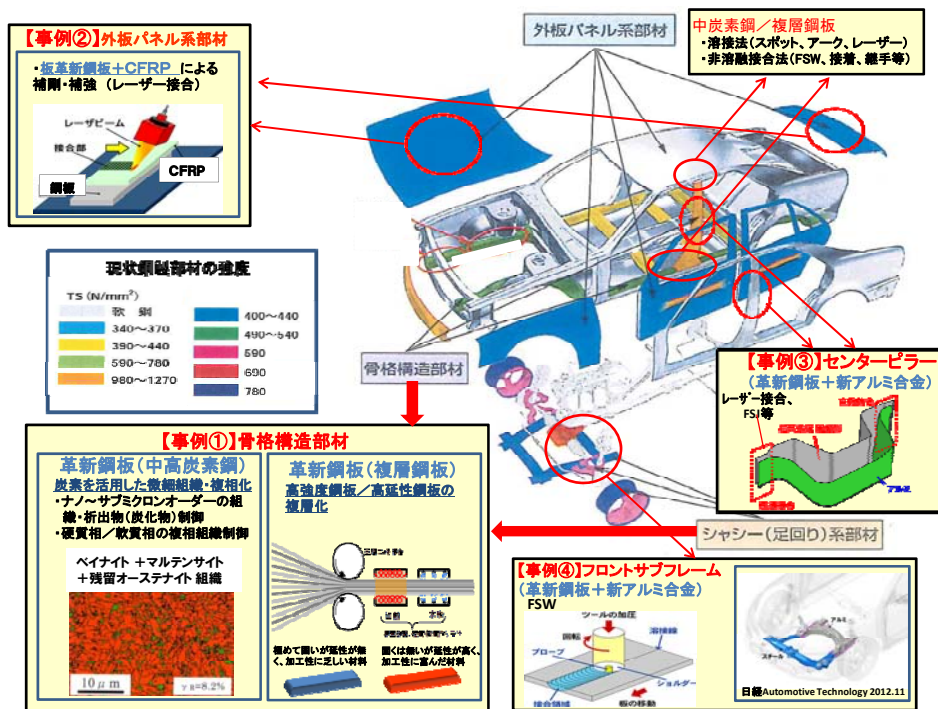
図1 自動車の材料構成と異種材料接合技術
