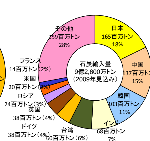
世界の石炭輸入量(2009年)
