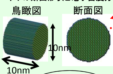
直径10nm(40,000原子)シリコン・ナノワイヤの断面形状と電子密度分布(例)
