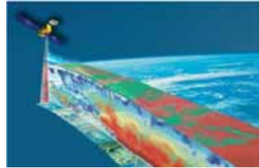
EarthCARE衛星イメージ図 雲とエアロゾルの3次元測定
