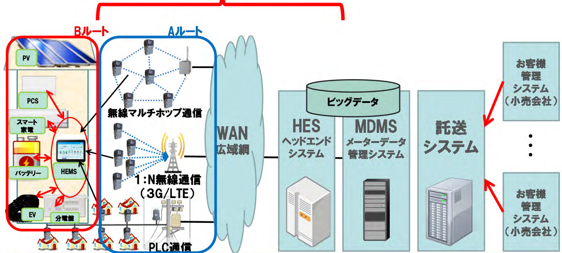
スマートメーター通信システム
