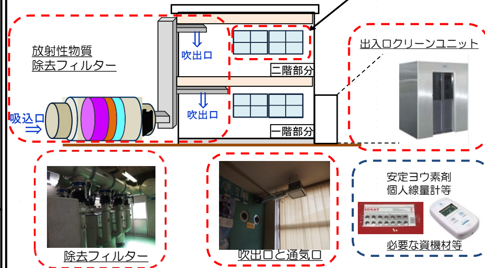
放射線防護対策のイメージ図
