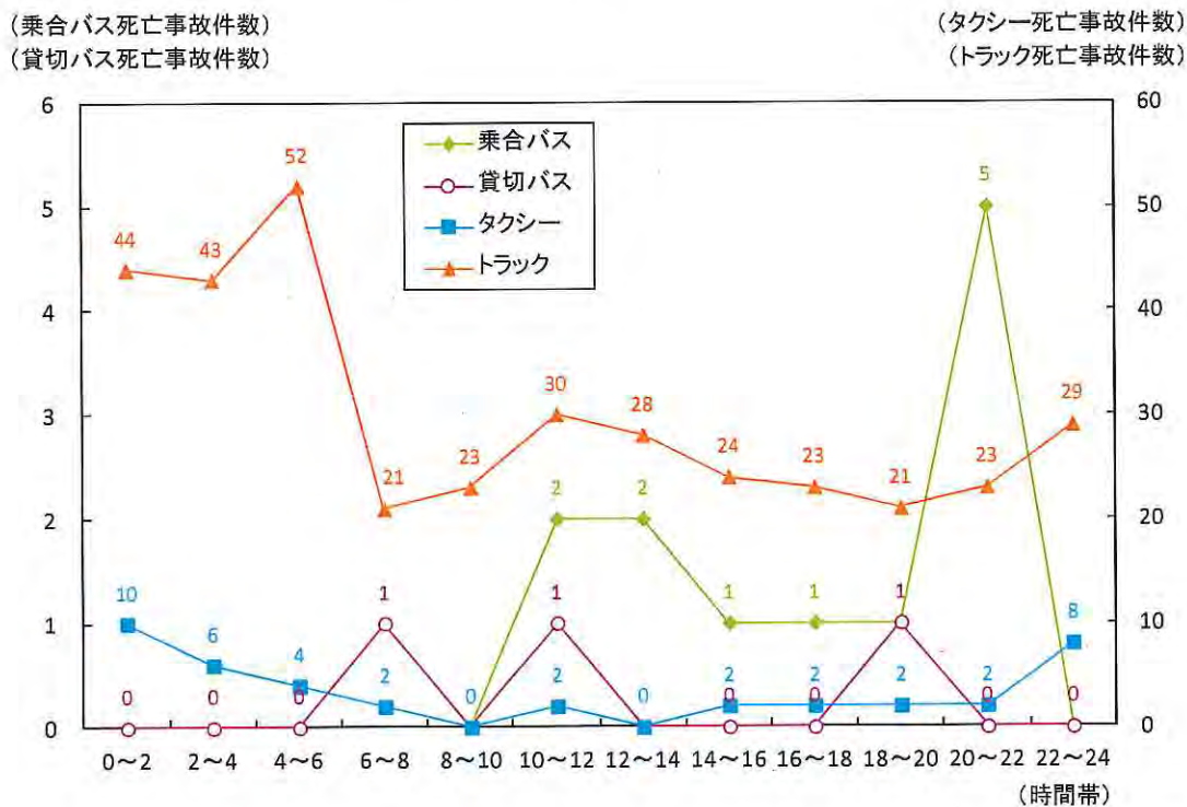
図 23 業態別時間帯別交通死亡事故件数 (平成25年)
