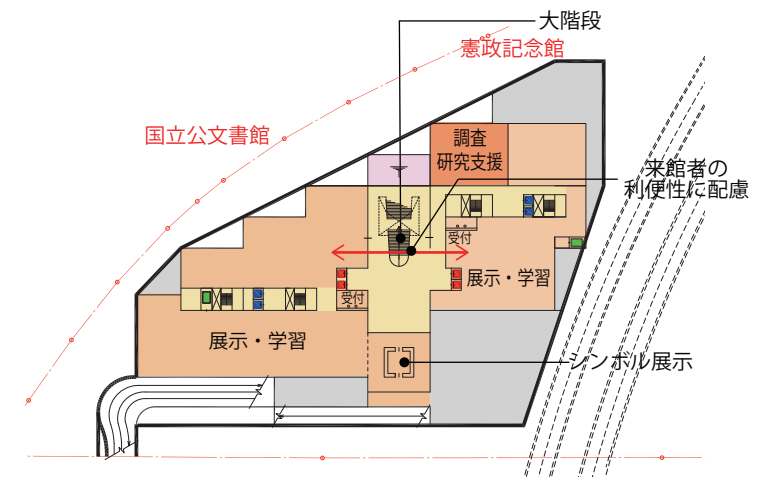
地下1階平面計画図
