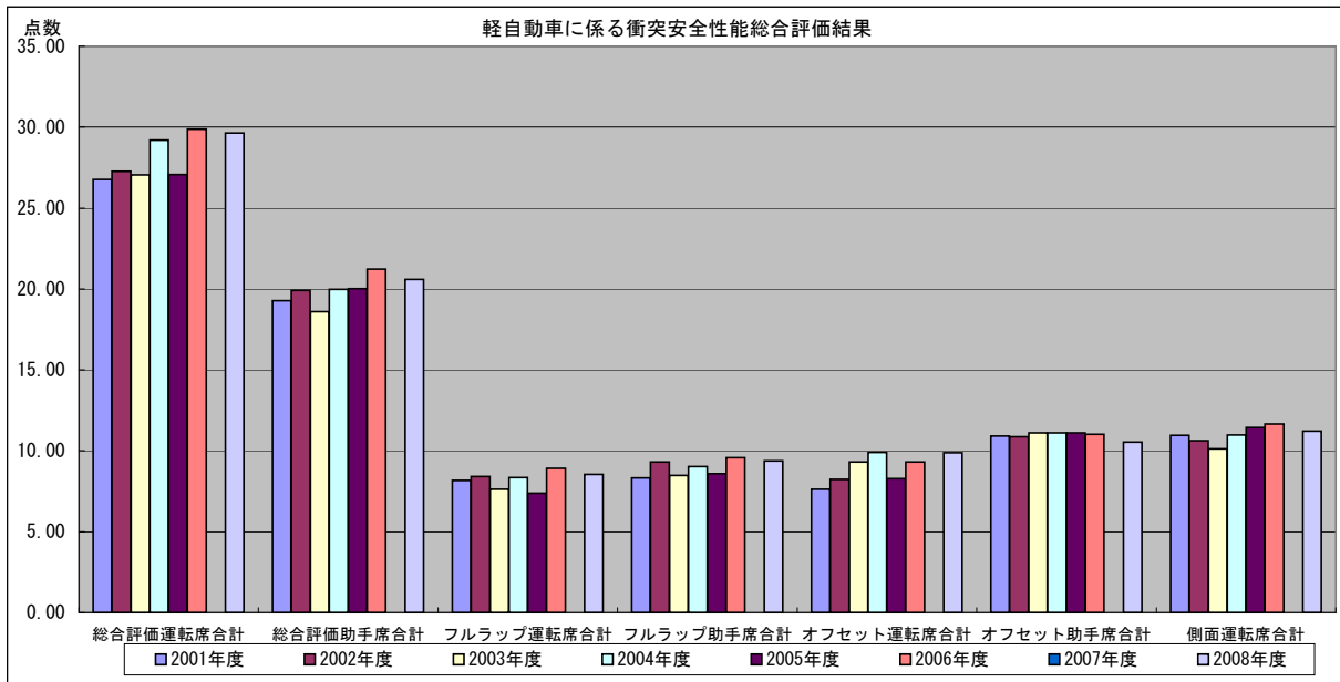
衝突安全性能総合評価結果(2001年度～2008年度)
