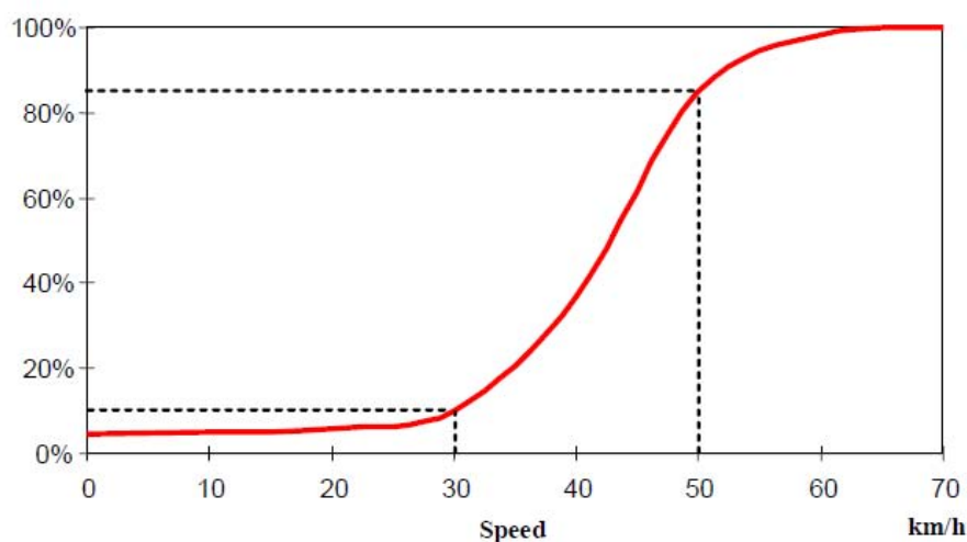
図6 車両に衝突された歩行者が死亡する確率
