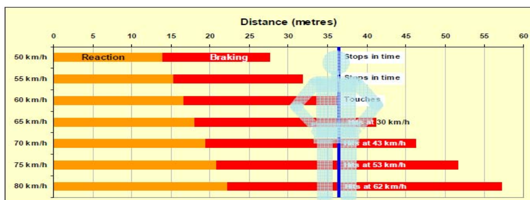
図1 速度による停止距離（1秒の反応時間を含む）
