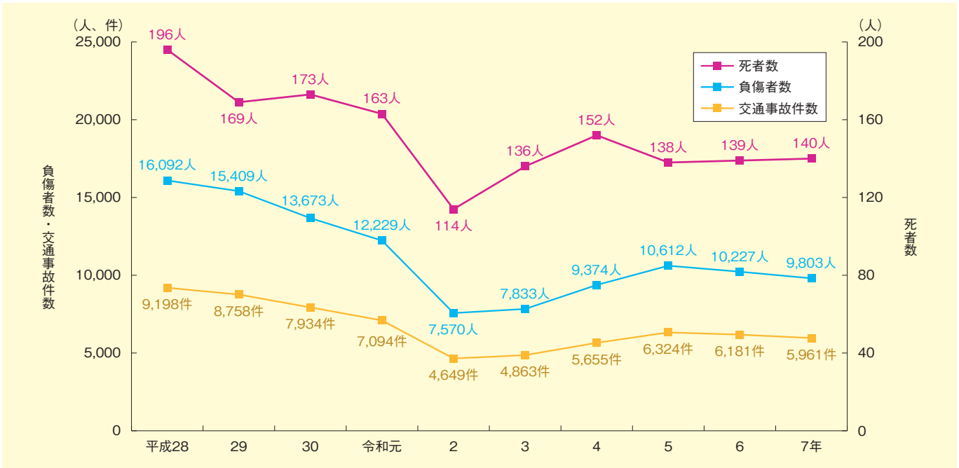
▶第1-27図 高速道路における交通事故件数、死者数及び負傷者数の推移
