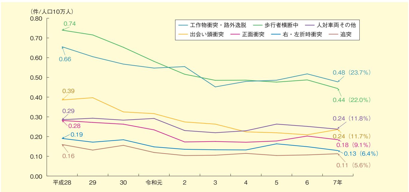
▶第1-4図 事故類型別人口10万人当たり交通死亡事故件数の推移
