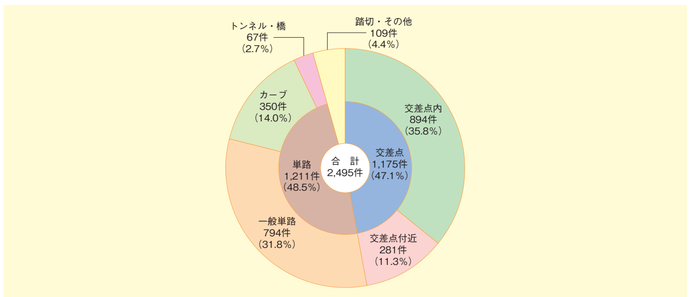
▶第1-14図 道路形状別交通死亡事故件数（令和7年）
