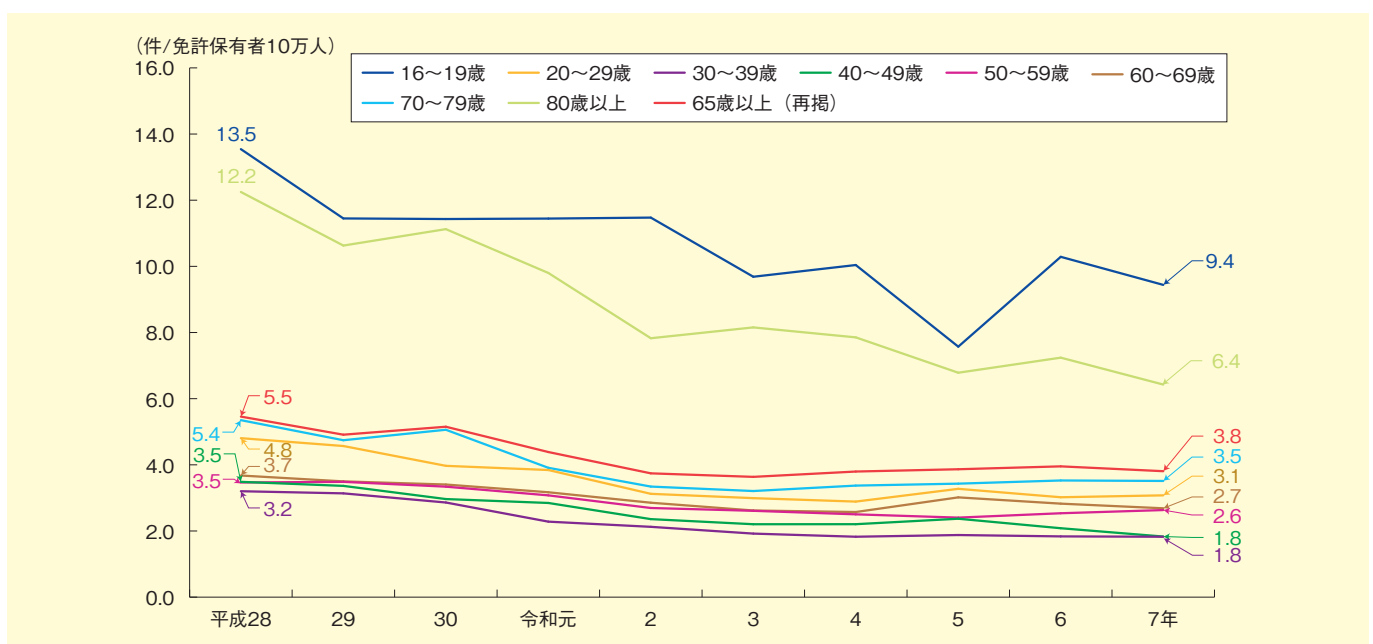
▶第1-15図 自動車、自動二輪車又は一般原付運転者（第1当事者）の年齢層別免許保有者10万人当たり交通死亡事故件数の推移
