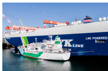
LNG バンカリング船「かぐや」 （提供：セントラルLNG マリンフューエル株式会社）
