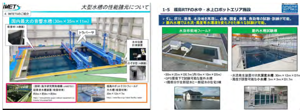
図 4-4 実験水槽の例（左図 防衛装備庁：岩国海洋環境試験評価サテライト大型水槽（IMETS）、右図 福島ロボットテストフィールド 水中・水上ロボットエリア施設）
