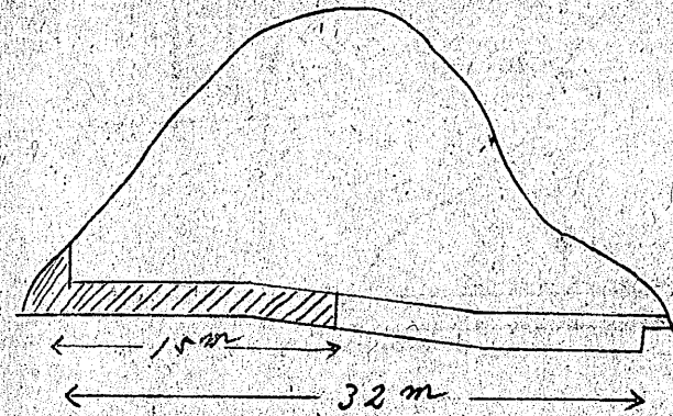
1.5 断面圖
