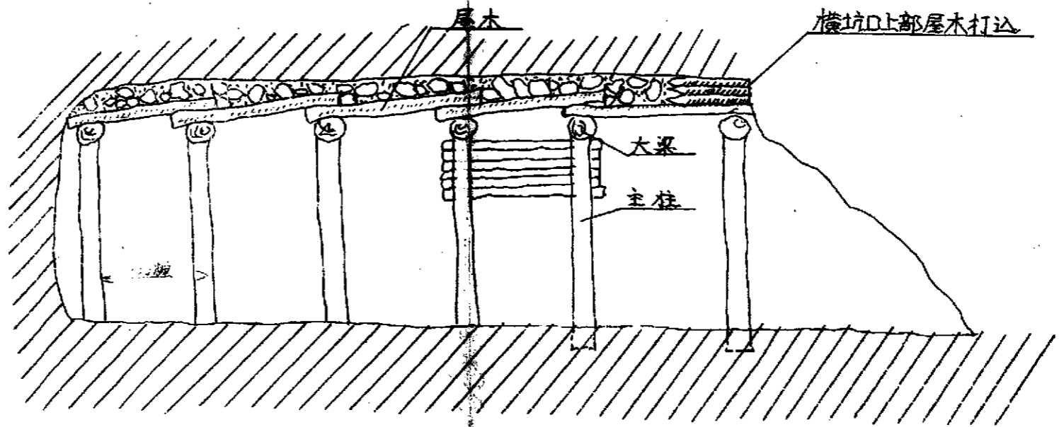
橫坑E-F縱斷面圖
