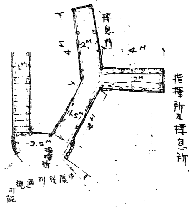
指揮班觀測所及指揮所棲息所計畫
