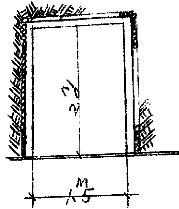
掩蔽部坑道断面 1/50
