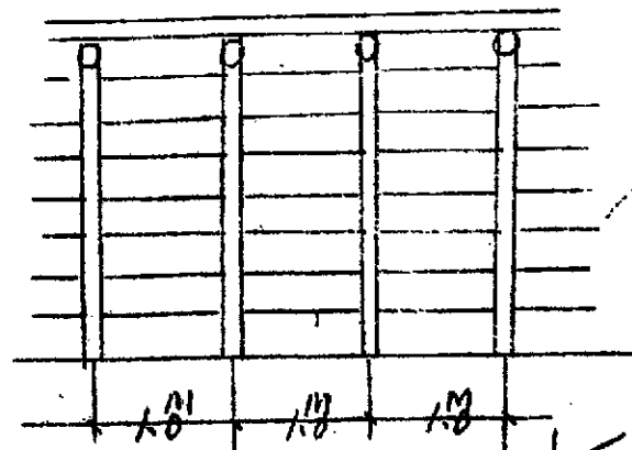
坑道縱断面 1/50
