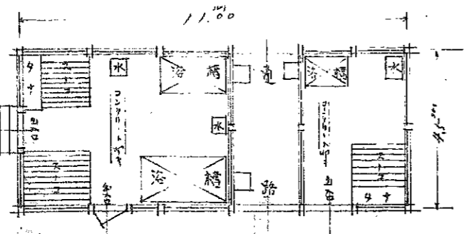
浴場平面圖
