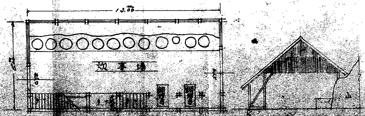
第三炮事場平面圖 正面圖 側面圖
