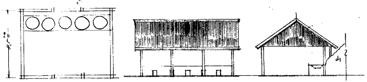
第一炮事場平面圖 正面圖 側面圖
