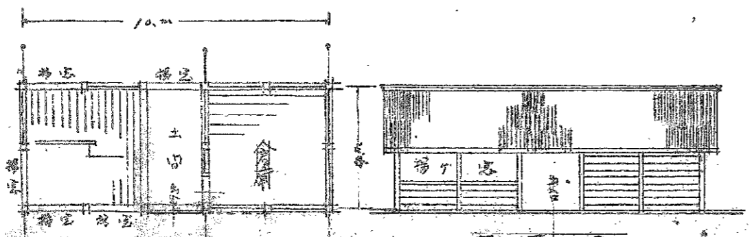
倉庫及倉庫設計平面图
