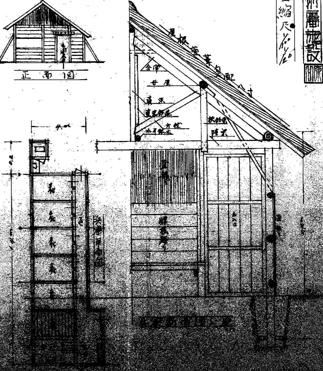
側面圖
