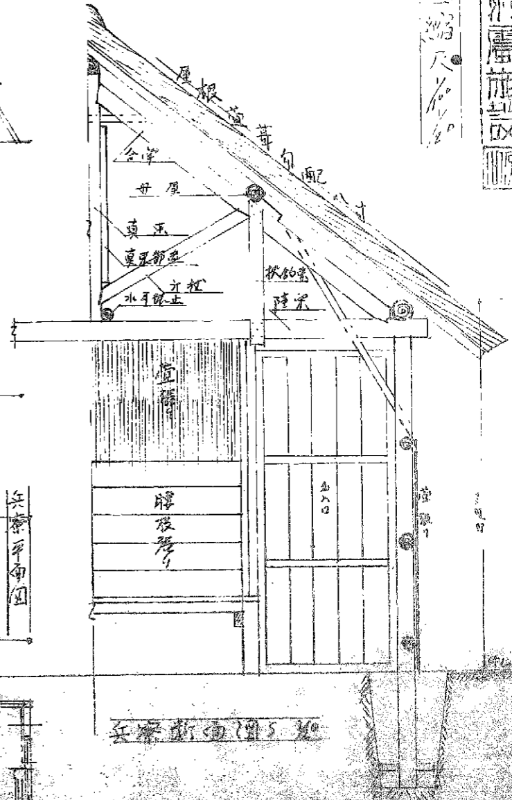
侧面图
