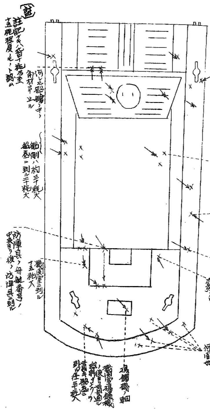
第七三二九號艇被害要圖
