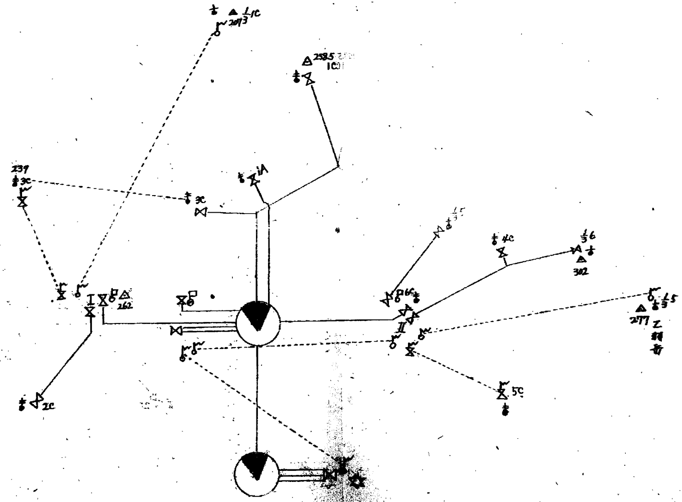
附圖第一 陣地内(戰國阿)通信網要圖
