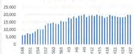
沖縄県の港湾取扱貨物量 (公共, 千トン)
