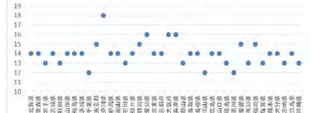
公共岸壁の都道府県別最大水深(m)
