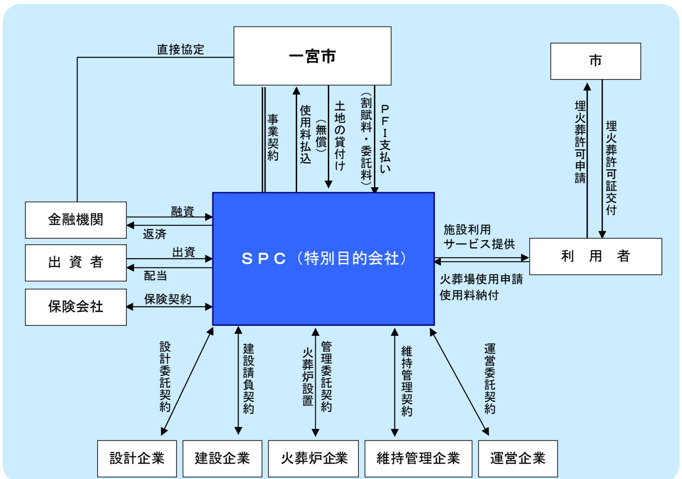
図 P F I 方式事業スキーム ( B T O 方式)
