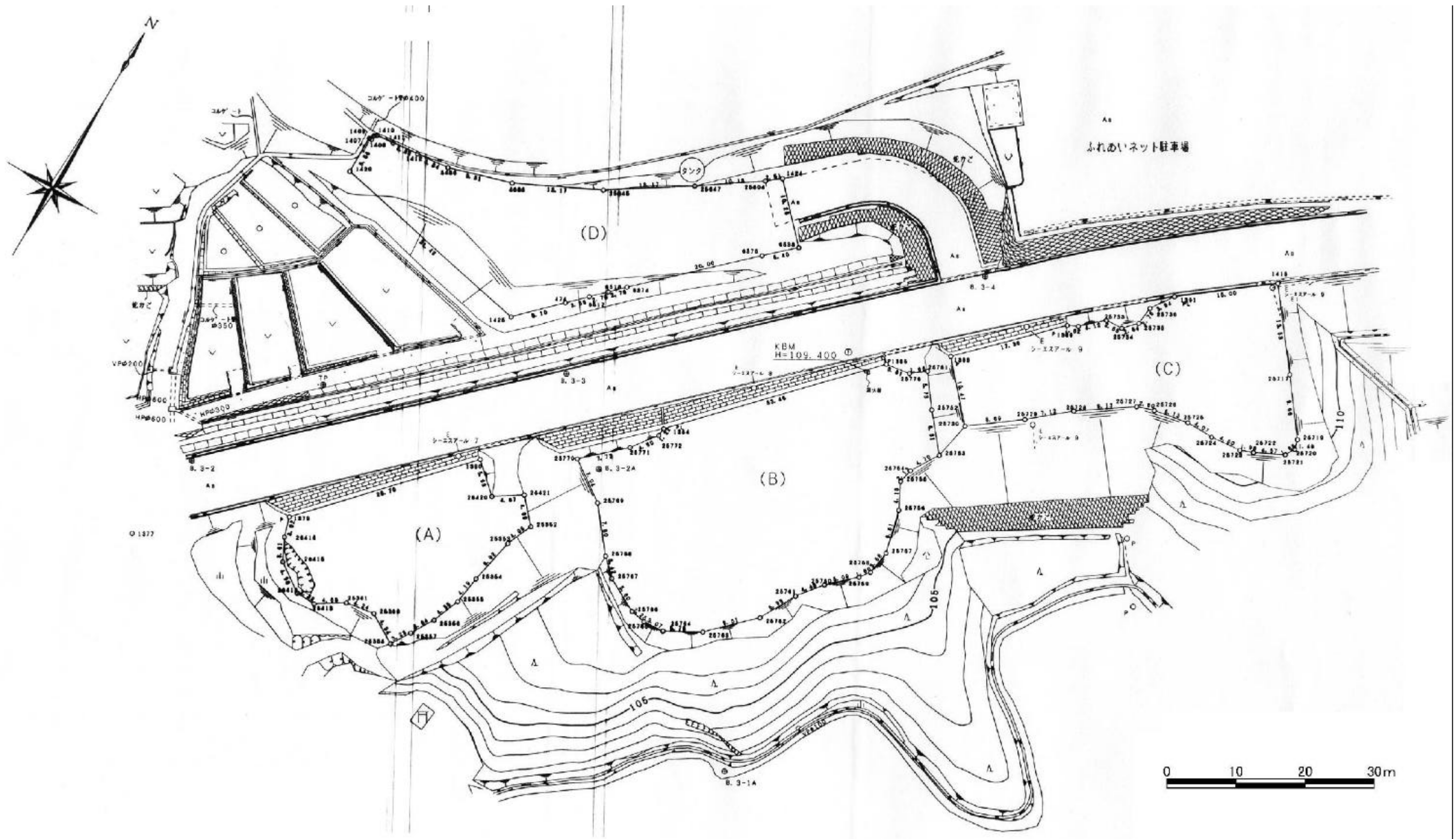
(2) 建設用地図面
