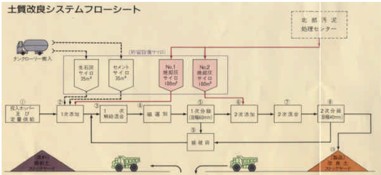
施設フロー図
