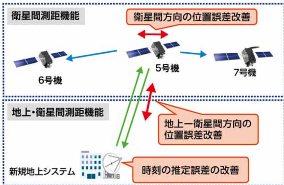
図 測位精度向上のための取組（衛星間測距、衛星/地上間測距を取り込んだシステム（高精度測位システム（ASNAV：Advanced Satellite NAVigation system））
