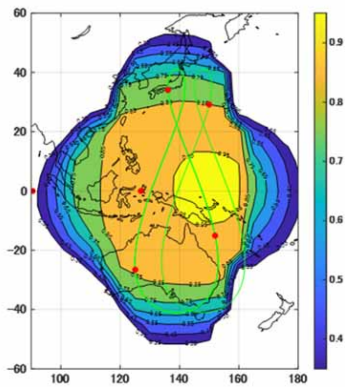
図 HDOP2.6 が得られる時間率分布の違いの目安(上:7機、下:11機)
