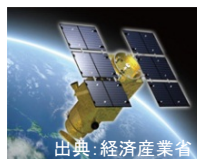
ASNARO-1
