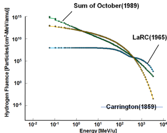
過去に起きたSPE(ワーストケース)のエネルギースペクトラム(ICRP123より)
