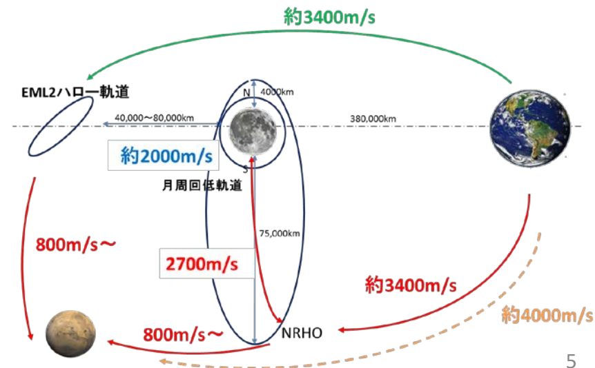
月周回拠点の軌道回りの概略増速量
