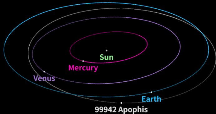
図1: Apophis軌道図
