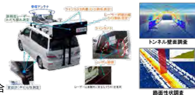
MMSによる道路形状等の取得
