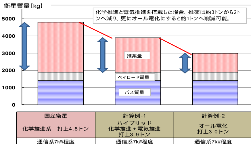
図 5：化学推進系と電気推進系の衛星重量比較
