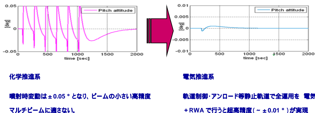
図 6：化学推進系と電気推進系の軌道位置制御精度の比較
