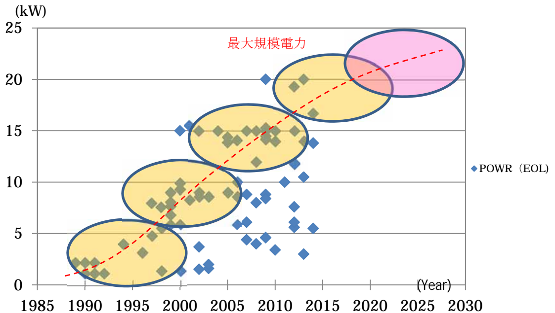
図 4 : 通信衛星電力の傾向分析
