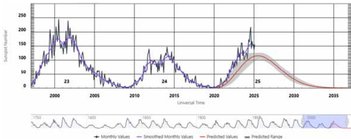
図 太陽活動の指標となる太陽黒点数の推移（NOAA の HP より）
