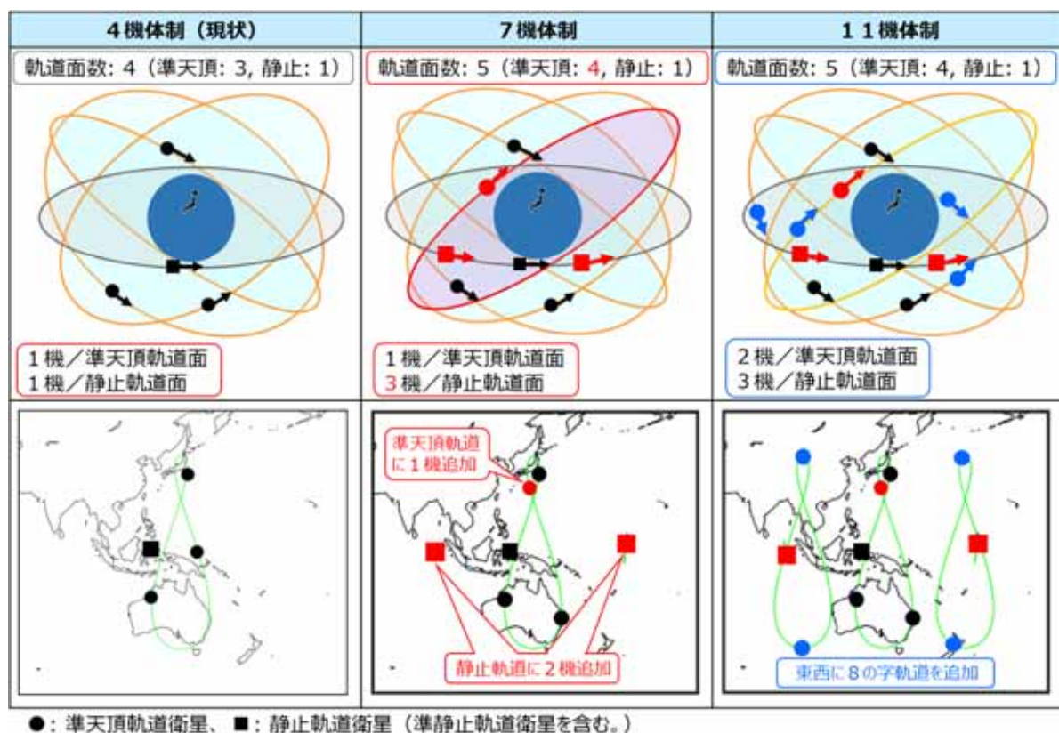
図 準天頂衛星システム「みちびき」の軌道追加、地上投影イメージ
